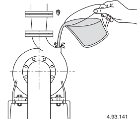
Fig. 8 Riempimento.
