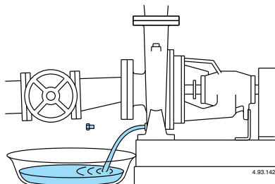
Fig. 9 Vidange.
