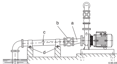
图4 管路连接
