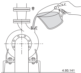
Abb. 8 Auffüllung.
