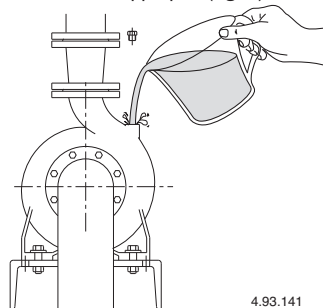
Fig. 8 Remplissage.
