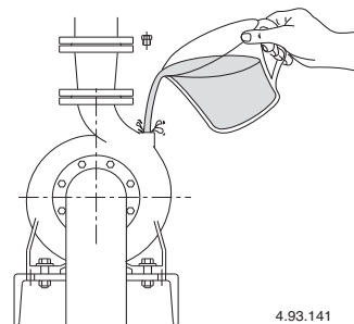
Bild 8 Fyllning.
