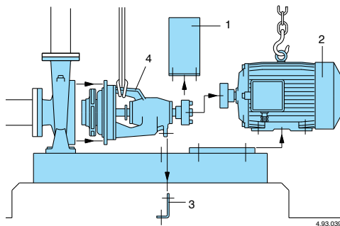
Fig. 10 Secuencia di smontaggio.
